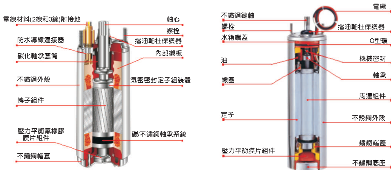
結構剖面圖
